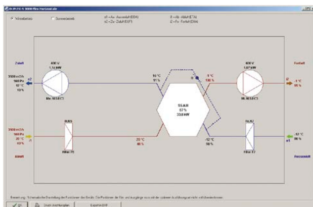
Funktionsplan
