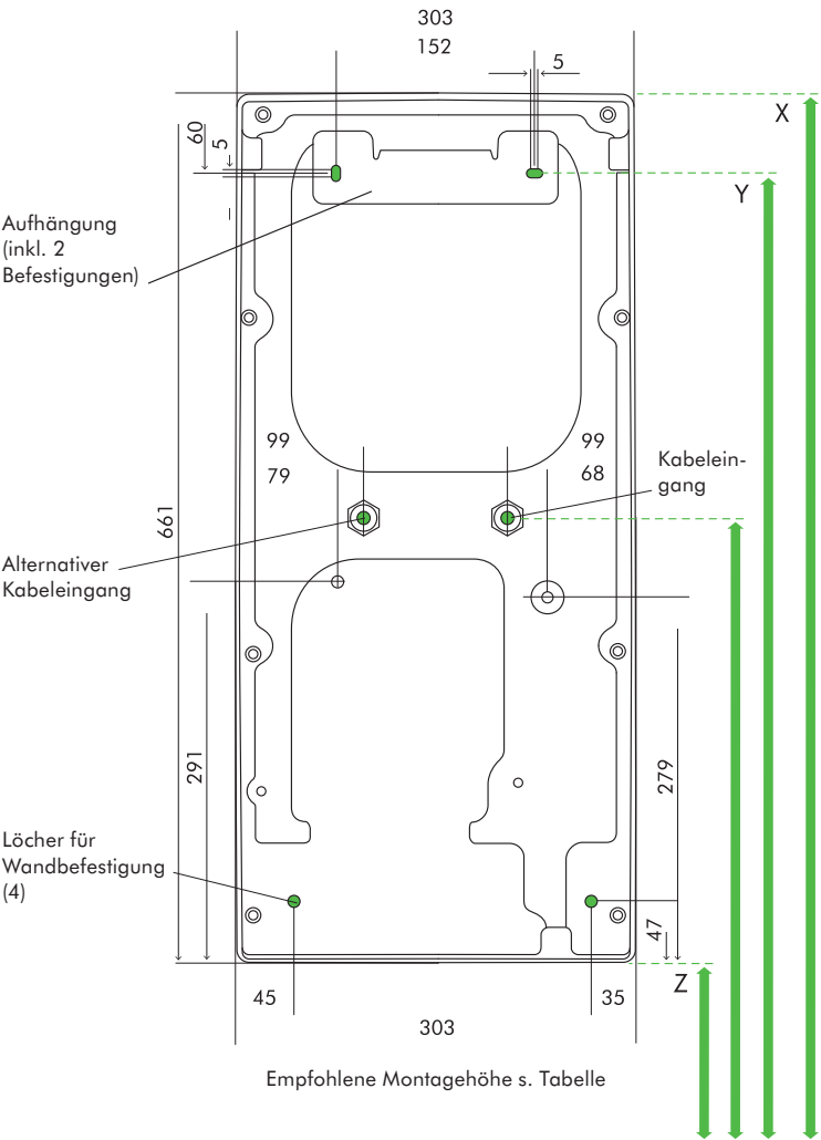
RÜCKANSICHT
