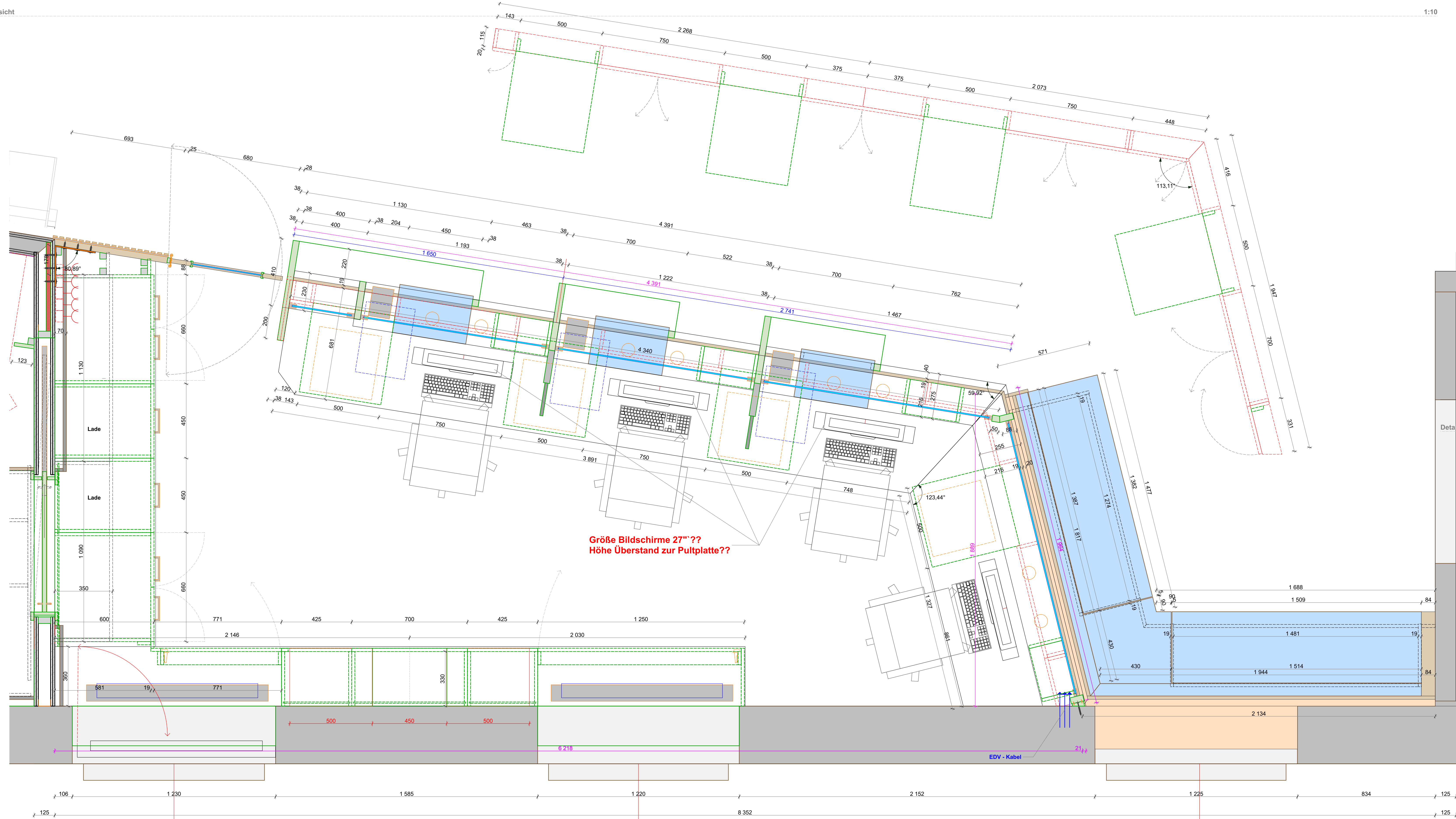
Grundriss
