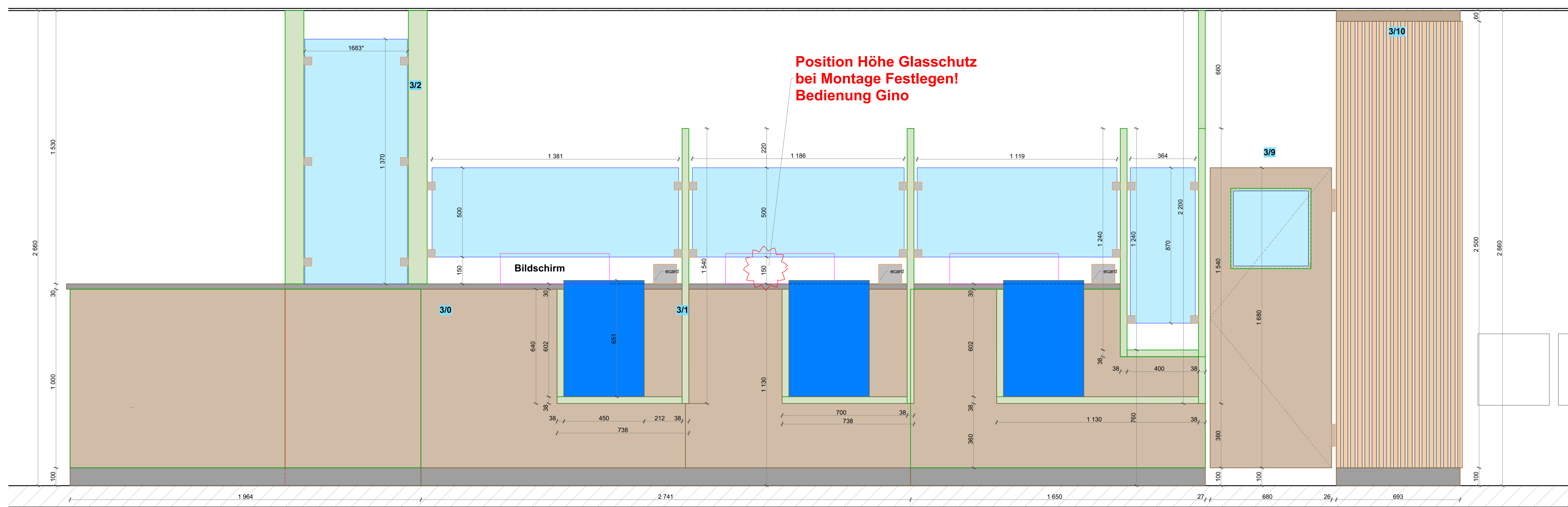
Ansicht
