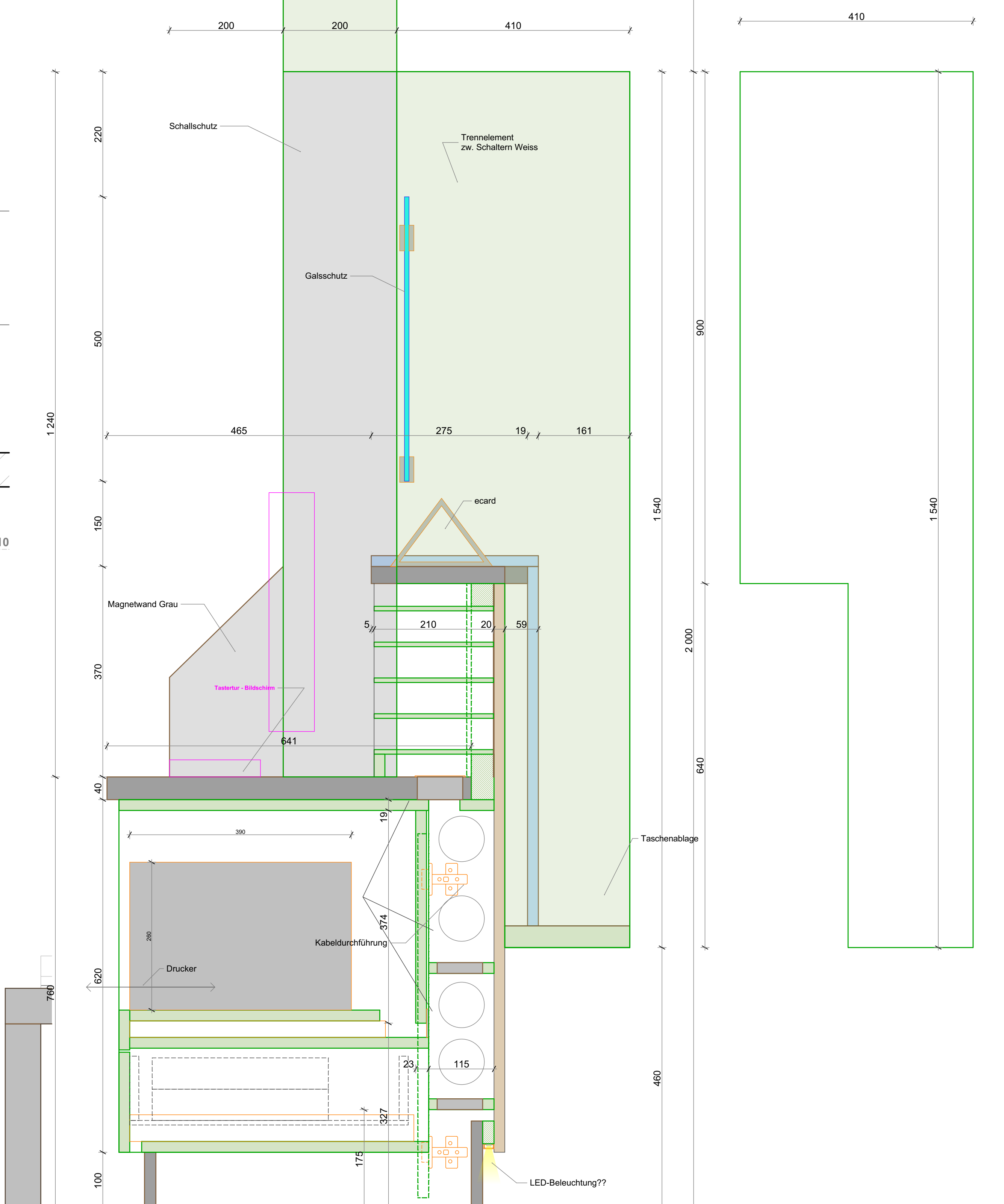
Detail Schnitt Empfangspult
